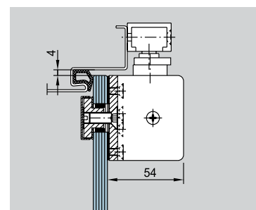
Dorma Befestigungsplatte für TS 92
