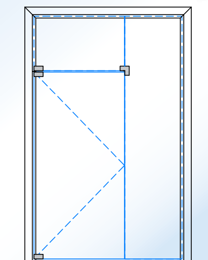
FZ 48 EA mit Oberlicht und Festverglasung Zargenprofil 3-seitig für Bodendrehlager bzw. BTS
