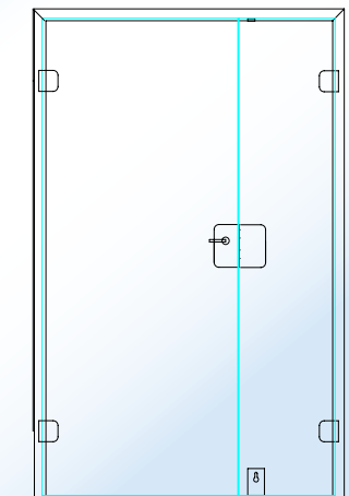
FZ 48 Typ C 1 flg. Türe mit Bedarfsflügel
