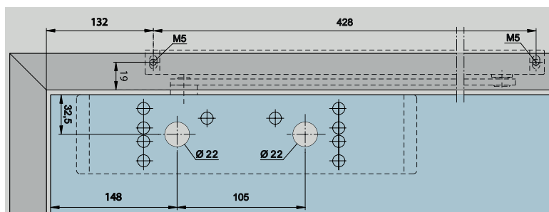
Dorma Obentürschließer TS 92 B, EN 1-4, für Studio/Junior
