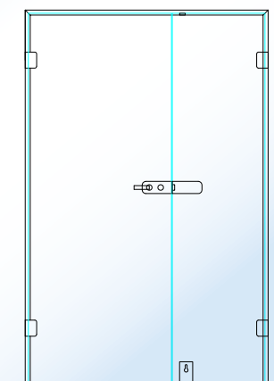
FZ 27 Typ C 1 flg. Türe mit Bedarfsflügel
