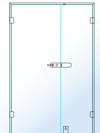
FZ 27 E Typ C 1 flg. Türe mit Bedarfsflügel
