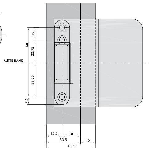
FZ 48 bei 8 mm Office M5 Gewindebohrung für Bandbefestigung
