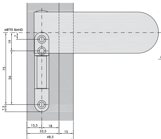
FZ 48 bei 8 mm Studio M5 Gewindebohrung für Bandbefestigung
