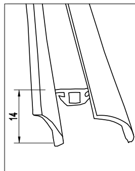
der ausgeklinkte Gummi muss oben im Querprofil durchlaufen
