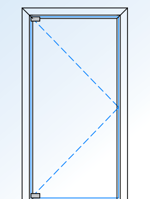
FZ 48 EA Zargenprofil 3-seitig für Boden- drehlager bzw. BTS
